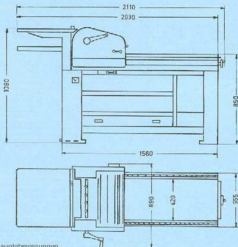
Hauptabmessungen
